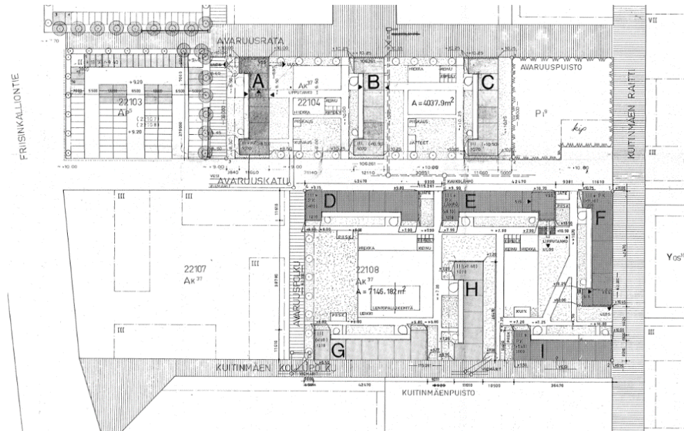
Kuva 8. Asemapiirros.
