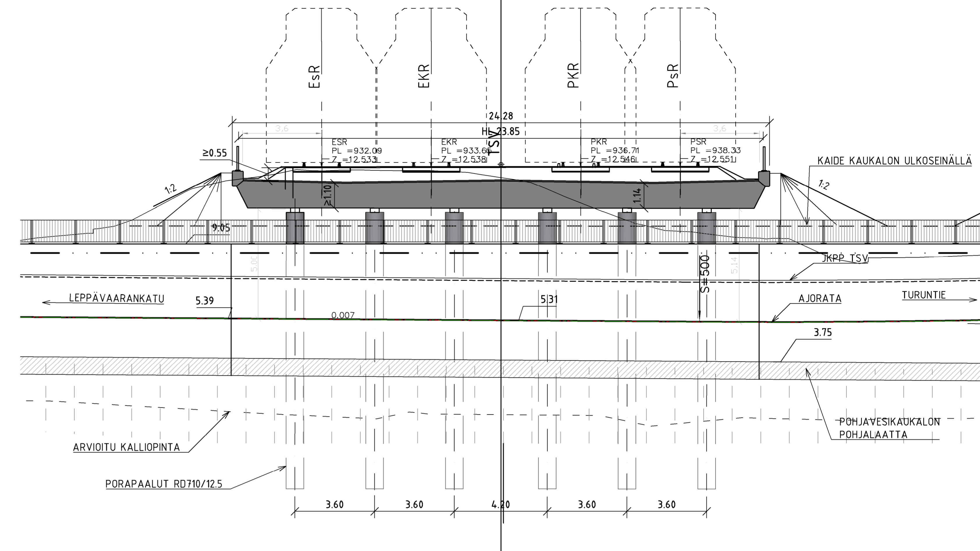
SILTAPAikka 1:5000
