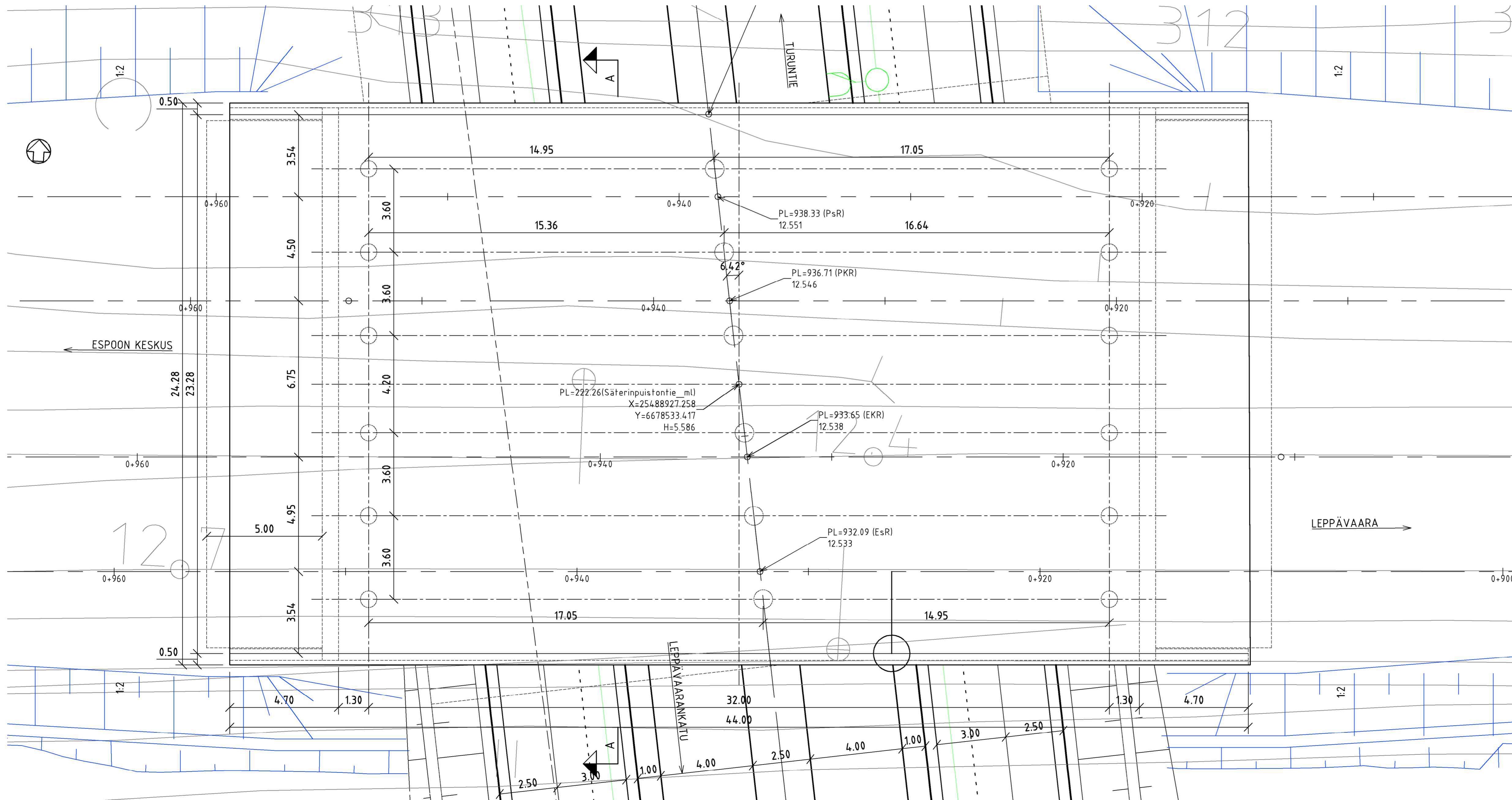
TASOKUVA 1:100
