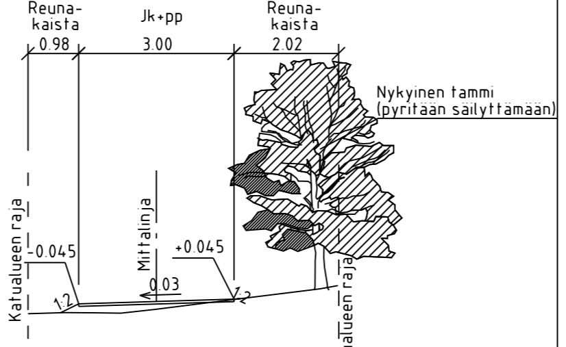
TYYPPIPOIKKILEIKKAUS B-B 1:100
