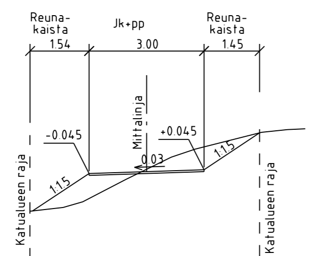
TYYPPIPOIKKILEIKKAUS A-A 1:100
