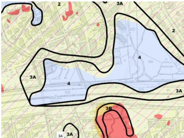
Kuva 21 Alueen maaperä- ja rakennettavuuskartta.
