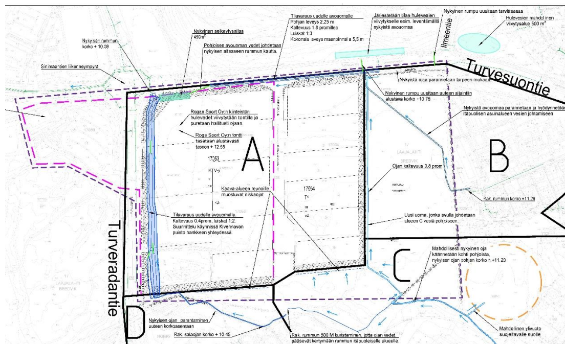
Hulevesisuunnitelman asemapiirros (3.11.2022).
