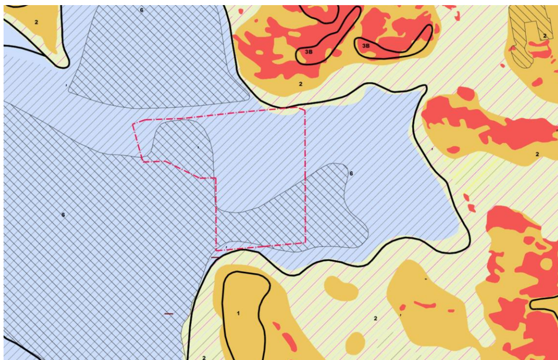
Maaperäkarta (3/2022)
