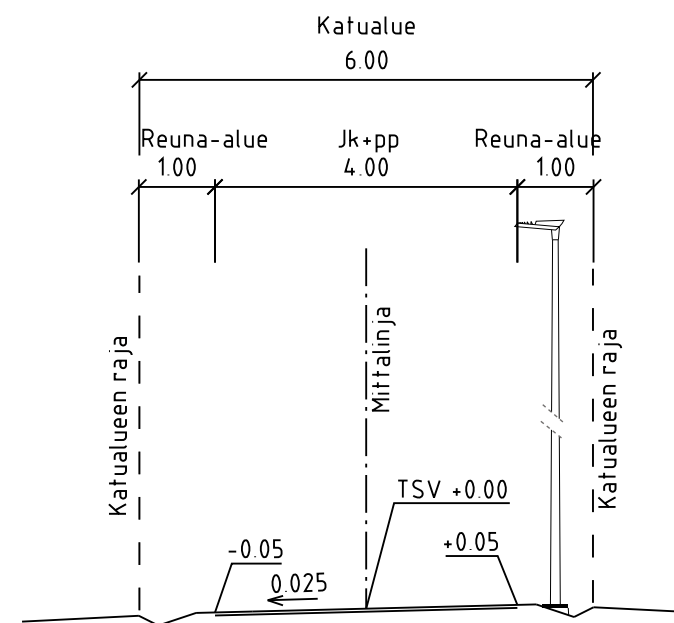
TYYPPIPOIKKILEIKKAUS A-A 1:100
