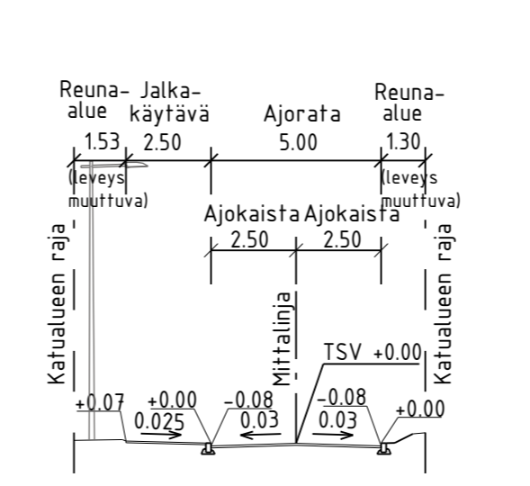
TYYPPIPOIKKILEIKKAUS B-B 1:200
