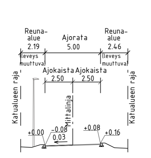
TYYPPIPOIKKILEIKKAUS A-A 1:200
