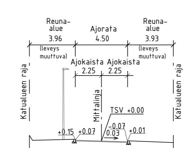
TYYPPIPOIKKILEIKKAUS A-A 1:200
