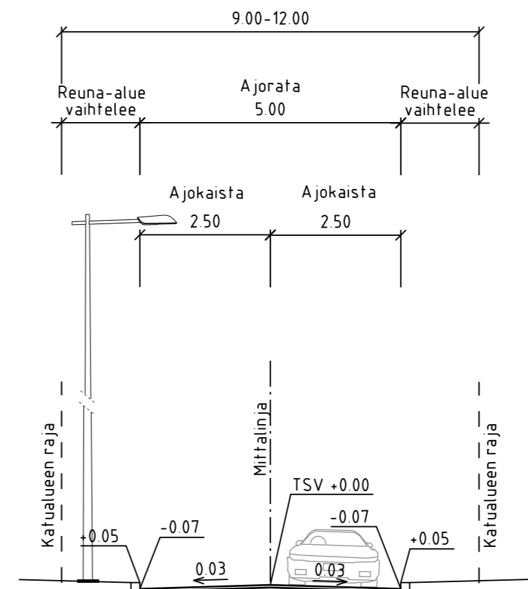
GOBBACKANRINNE TYYPPIPOIKKILEIKKAUS A-A 1:100
