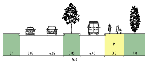
SÄTERINSOLMU (ramppi), LEIKKAUS C - C
