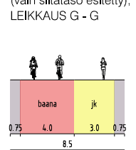
LAAJALAHDENBAANA (vain siltataso esitetty), LEIKKAUS G - G
