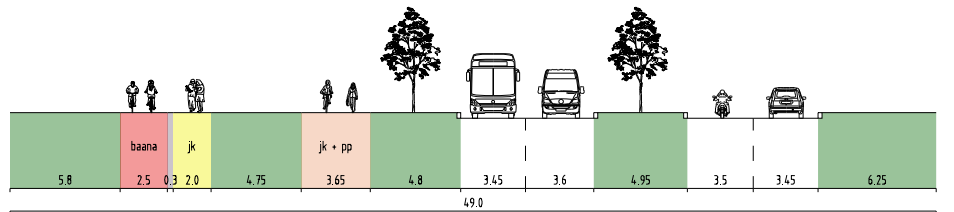
SÄTERINKATU, LEIKKAUS B - B
