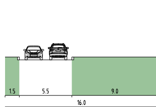
LUUTNANTINKATU, LEIKKAUS E - E
