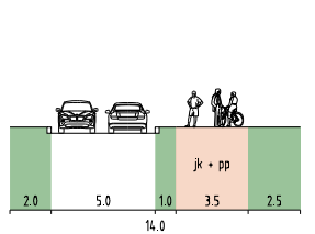
LUUTNANTINKUJA, LEIKKAUS D - D
