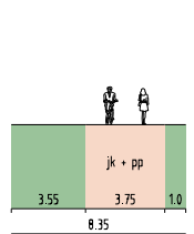
MAJURINPOLKU, LEIKKAUS F - F
