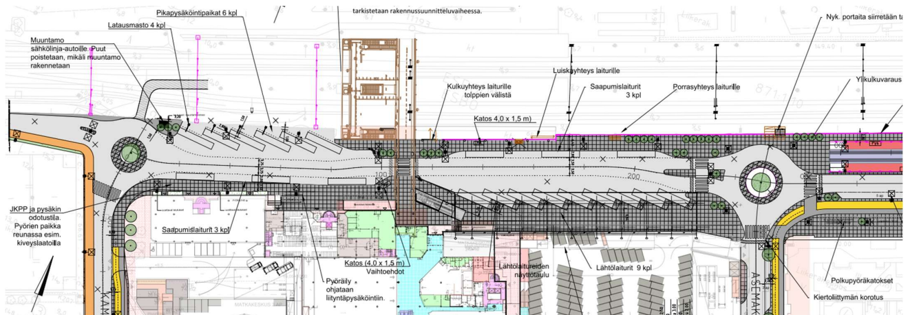
Kuva 30. Ote ktys-suunnitelmasta joukkoliikenneterminaalin alueelta.
