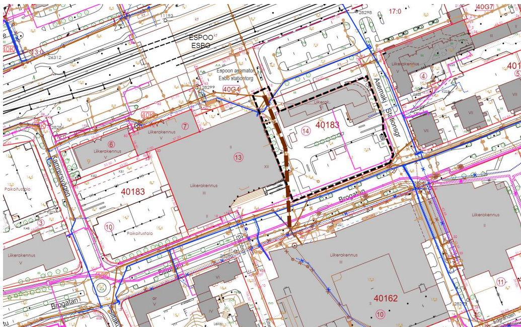
Kuva 11. Ote johtokartasta. Johtokartasta on nähtävissä tontin 14 (mustan katkoviivan mukainen alue) läpi kulkeva jätevesiviemäri (kuvassa ruskea katkoviiva).
