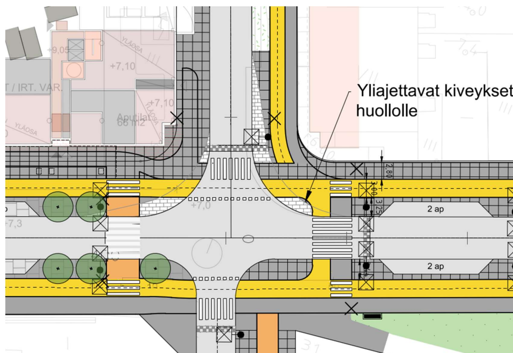
Kuva 29. Ote ktys-suunnitelmasta Asemakujan, Siltakadun ja Valakujan risteyksestä.
