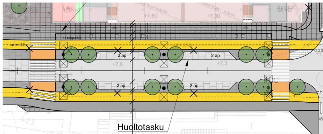
Kuva 28. Ote ktys-suunnitelmasta Siltakadun itäosasta.
