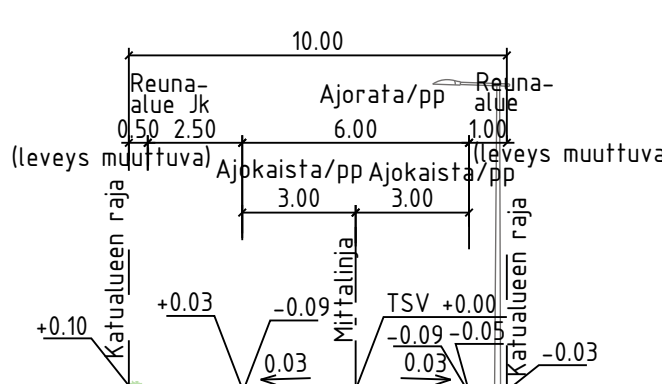
TYYPPIPOIKKILEIKKAUS B-B 1:200
