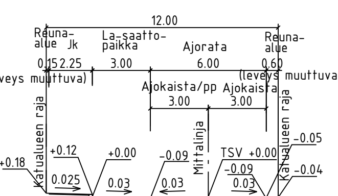
TYYPPIPOIKKILEIKKAUS A-A 1:200
