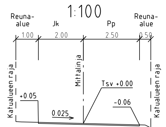
TYYPPIPOIKKILEIKKAUS A-A
