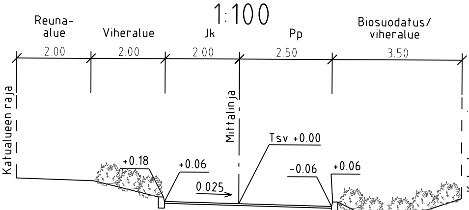
TYYPPIPOIKKILEIKKAUS B-B
