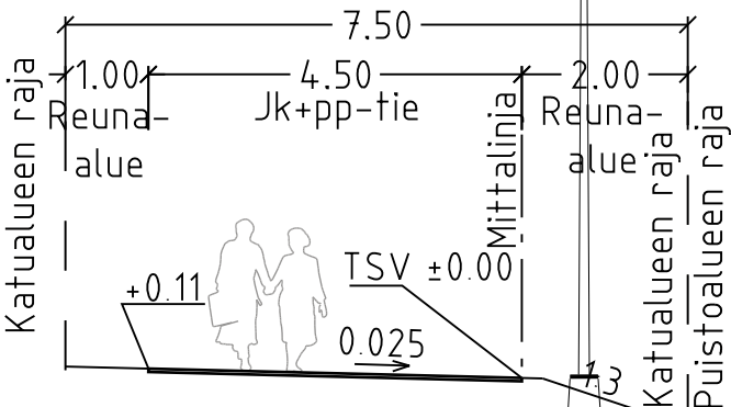
TYYPPIPOIKKILEIKKAUS A-A 1:100
