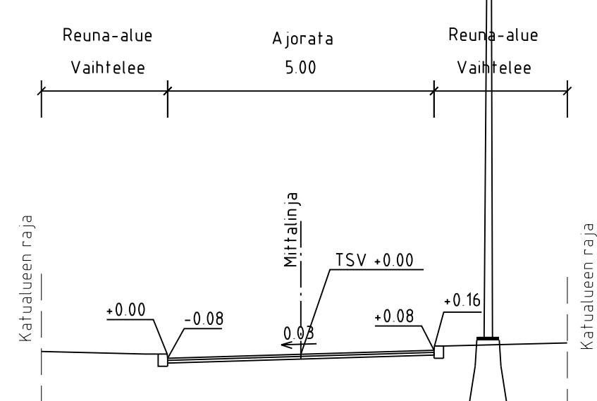
VALSSIKUJA TYYPPIPOIKKILEIKKAUS B-B 1:100
