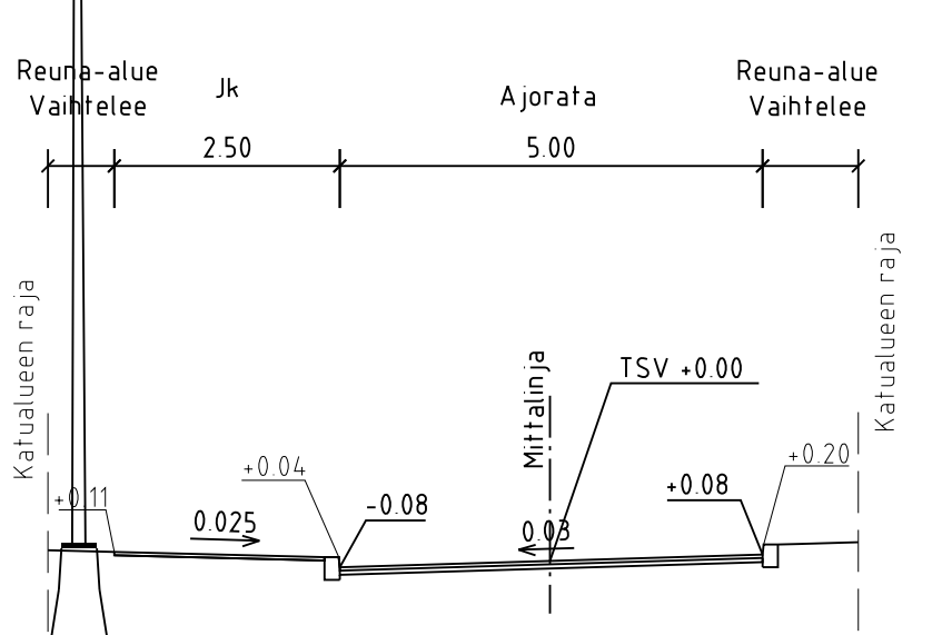
VALSSITIE TYYPPIPOIKKILEIKKAUS C-C 1:100
