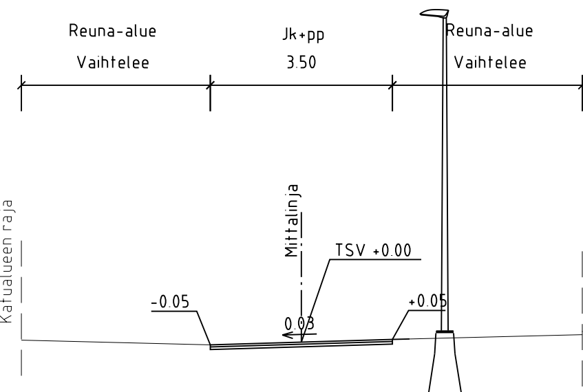
VALSSIKUJA TYYPPIPOIKKILEIKKAUS A-A 1:100
