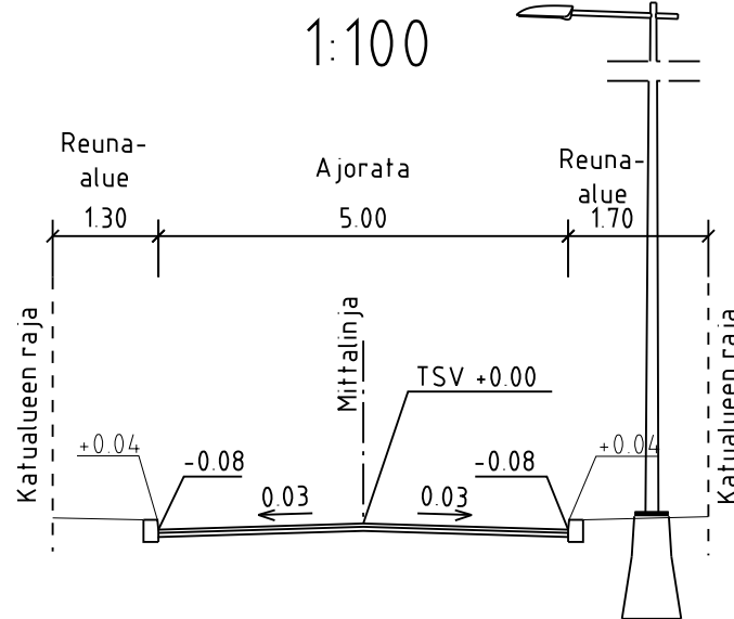
TANGOKUJA TYYPPIPOIKKILEIKKAUS B-B 1:100
