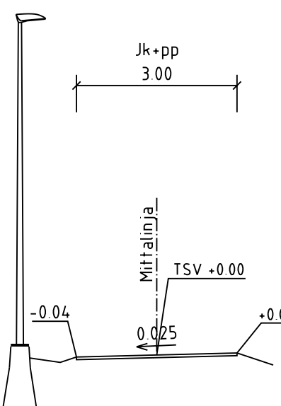
RAITTI 1 TYYPPIPOIKKILEIKKAUS C-C 1:100
